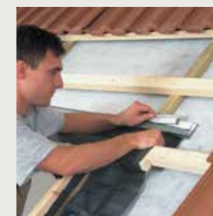
Посилений дренажний жолоб, який не потребує додаткової опори
